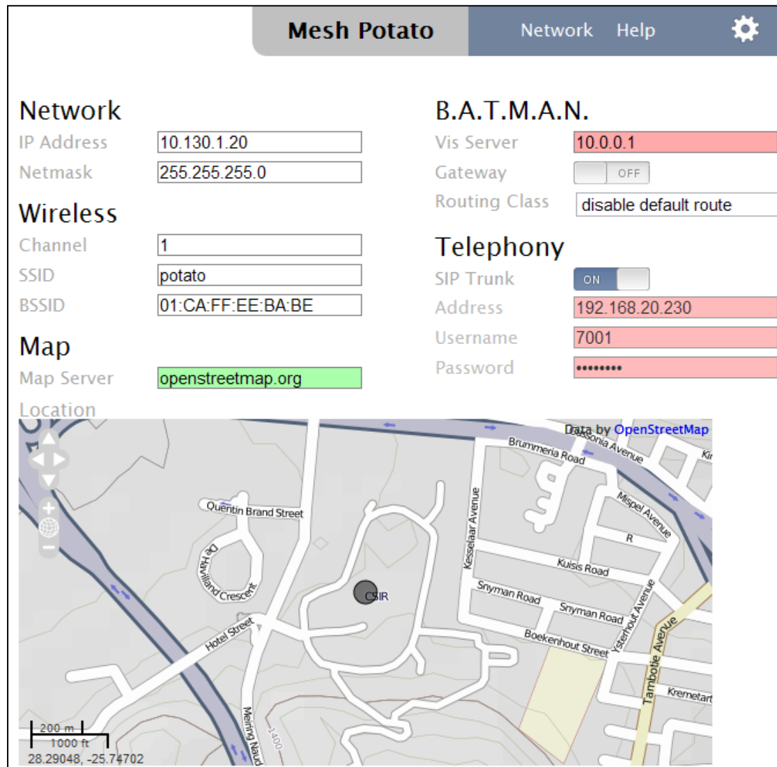
Mesh Potato GUI
